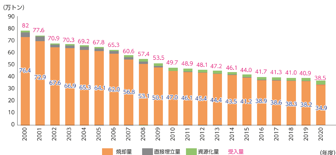
図4 2020年度までの本市のごみ量の推移
