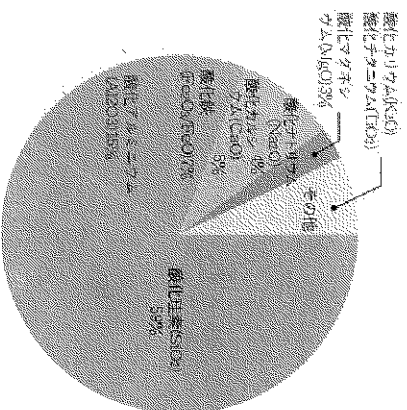
火成岩の構成
