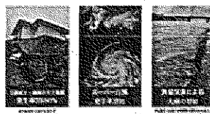
日本の自然災害の発生件数・被害は この数十年増加傾向
