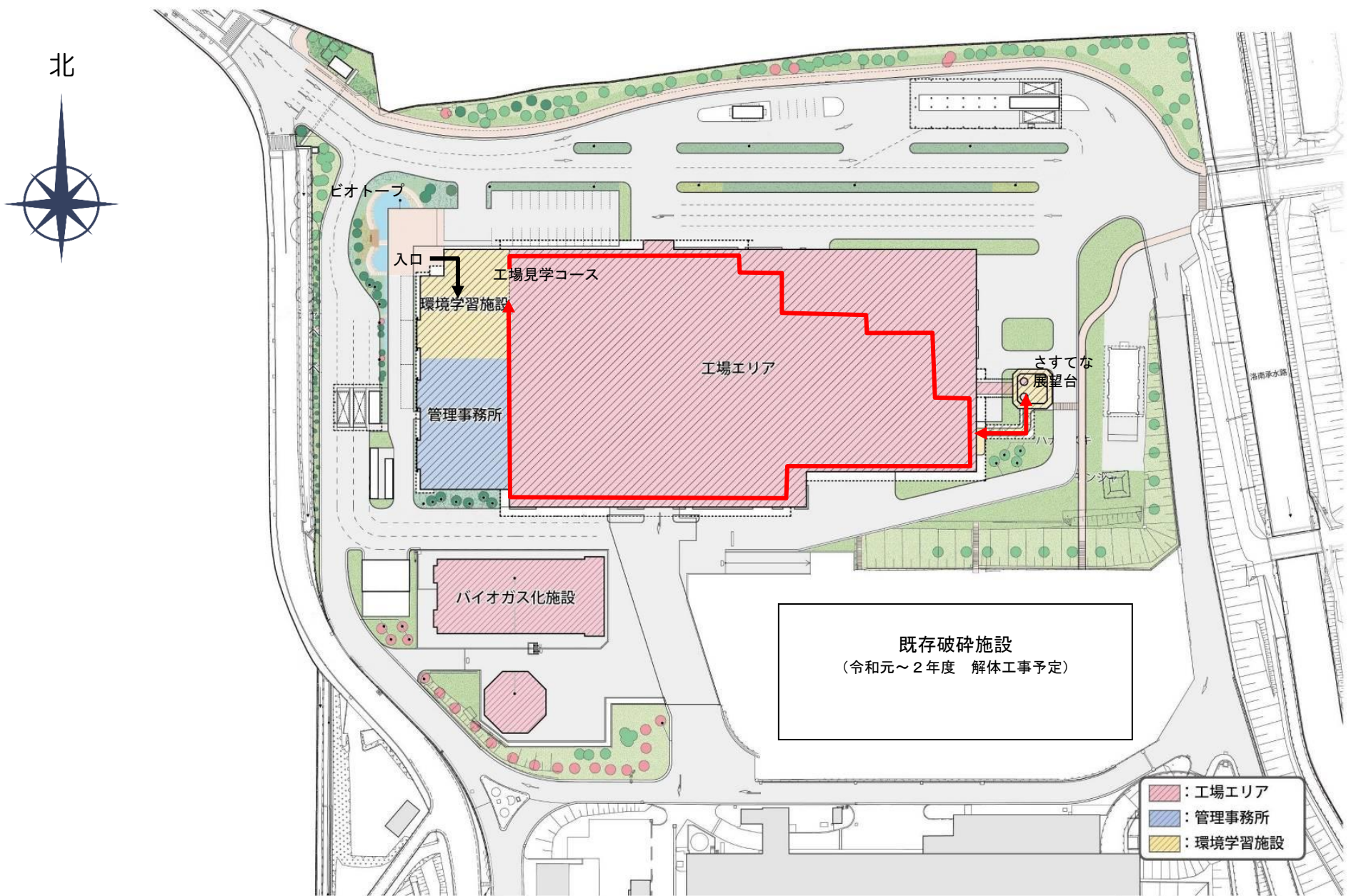
第二工場配置図
