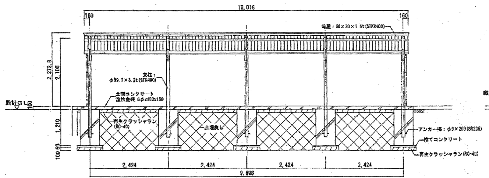
職員用駐輪場 2 正面図
