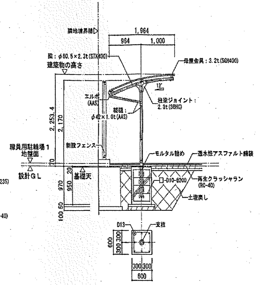
職員用駐輪場 1 側面図
