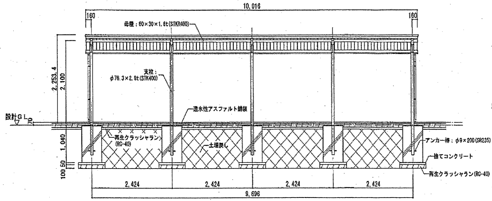
職員用駐輪場 1 正面図
