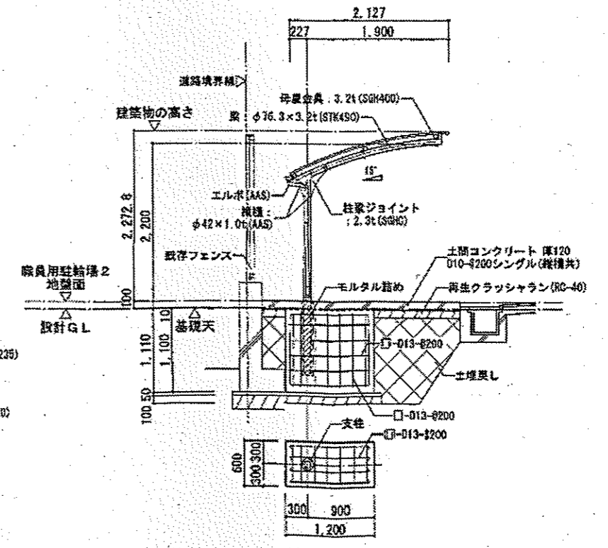
職員用駐輪場 2 側面図
