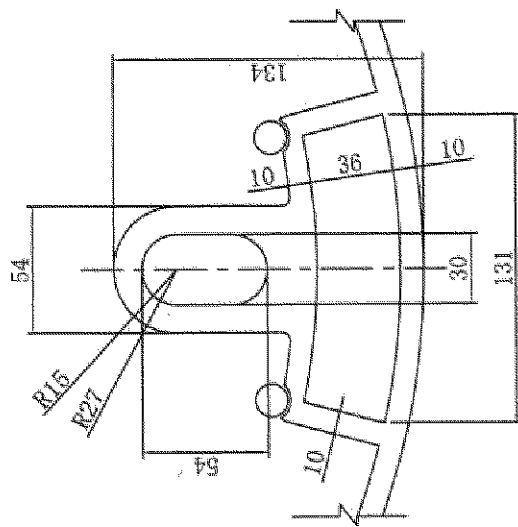
カギ穴及び文字座詳細図
