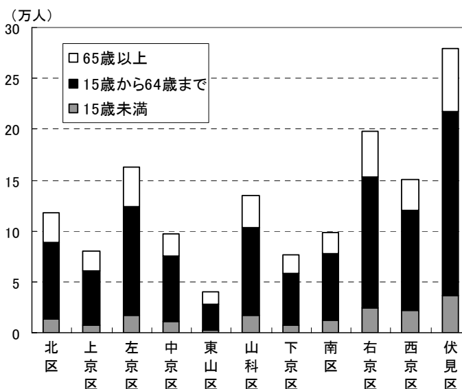
図-2 京都市の行政区別年齢3区分別人口(年齢不詳を除く。)
